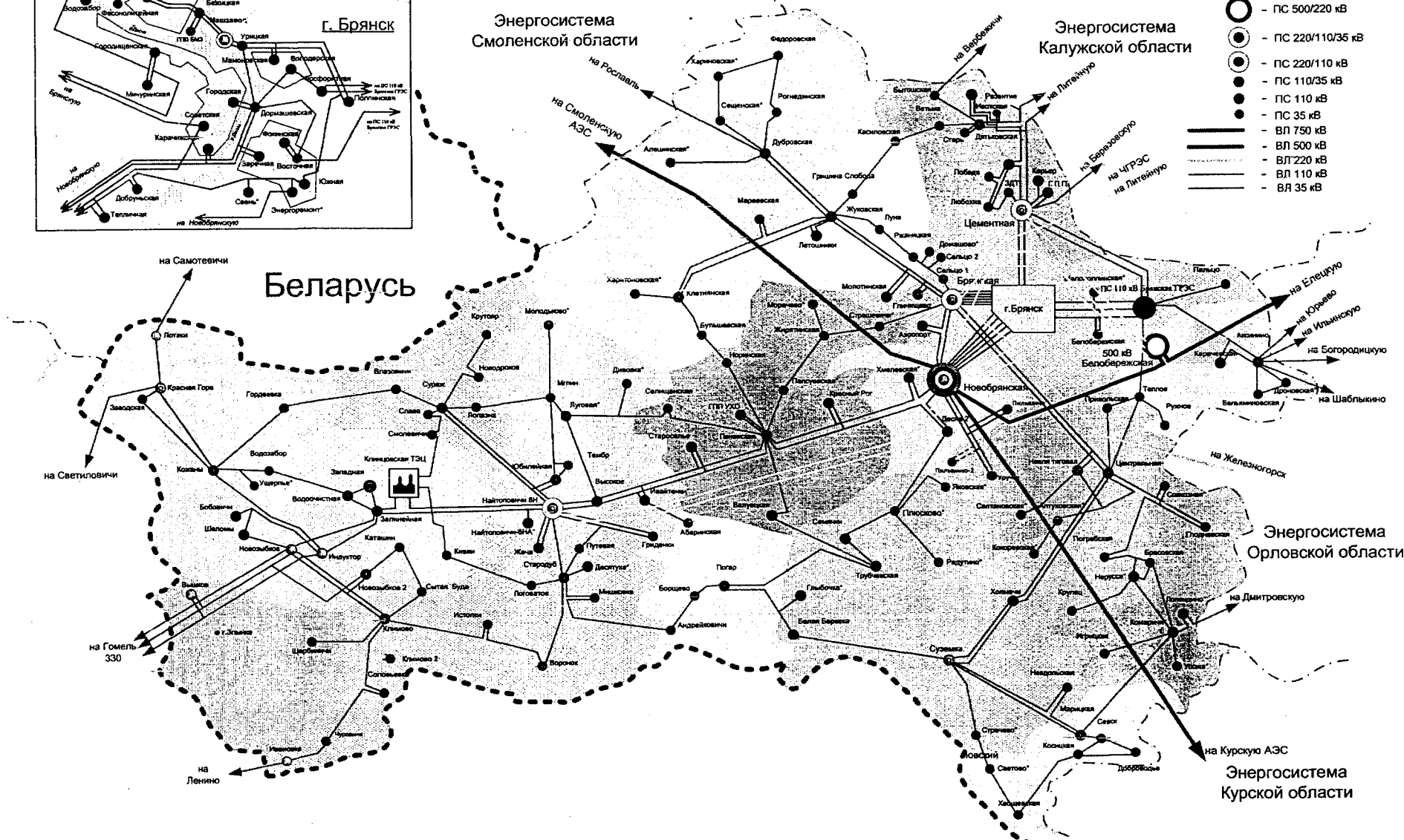
Схема развития электроэнергетики Брянской области на 2023 - 2027 гг.
