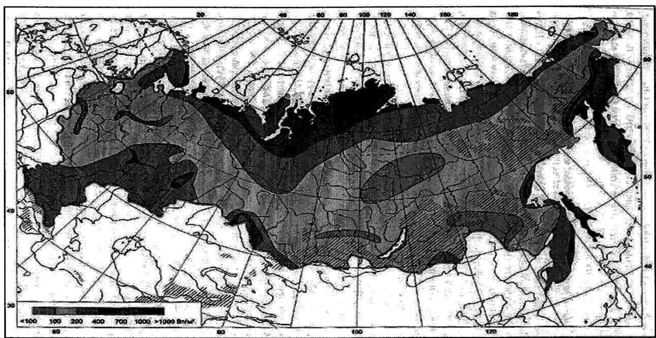
Рисунок 10. Распределение удельного ветропотенциала ( Вт/м^2 ) на высоте 100 м
