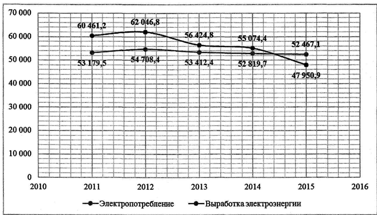
Рисунок 6. Баланс электрической энергии ЭС Иркутской области, млн. кВт. ч
