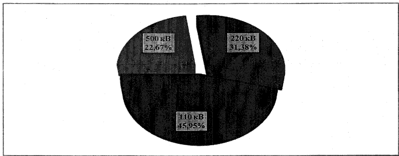
Рисунок 7. Структура протяженности ВЛ и КЛ по номинальному напряжению
