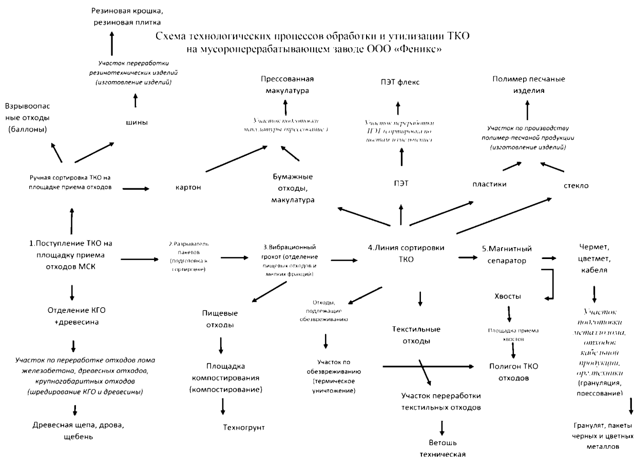
Рис 7.1. Схема технологических процессов обработки и утилизации ТКО на мусороперерабатывающем заводе ООО «Феникс»
