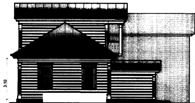
Восточный фасад.
