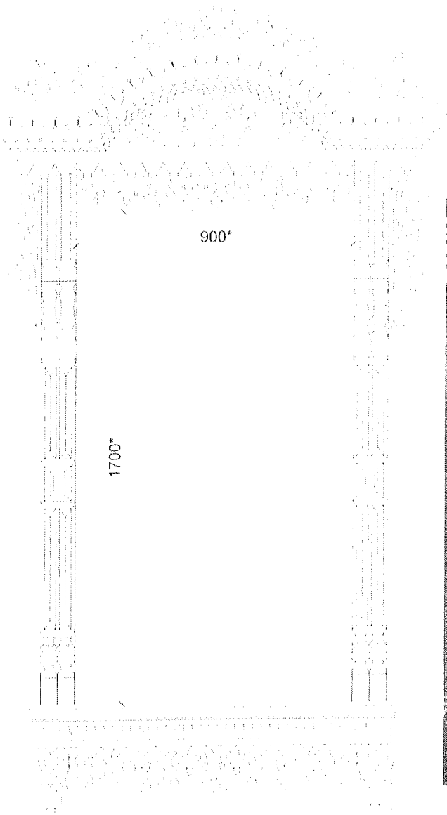
Рисунок 1. Резной наличник на 2-м этаже. М1:20.
