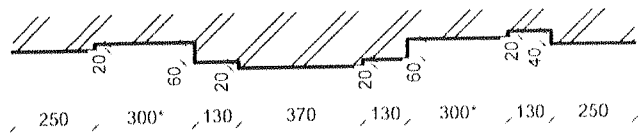
Сечение1. Рельефный декор из кирпича. М 1:20.
