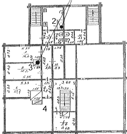
Местоположе ние печей на 2-м этаже.
