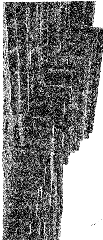
Сечение1. Рельефный декор из кирпича. М 1:20.
