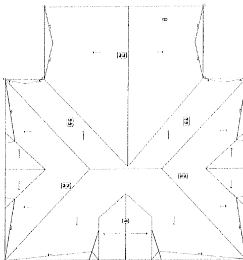
Схема кровли
