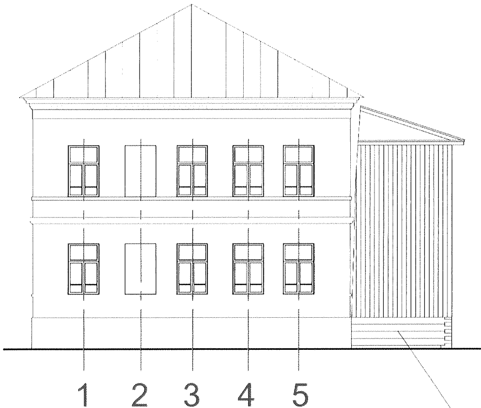
Южный фасад
