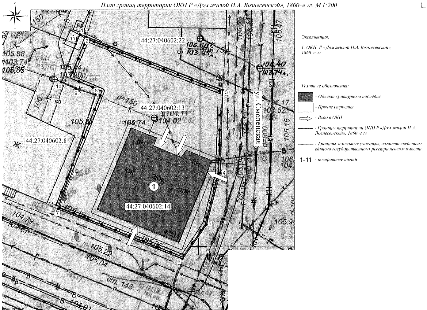
План границ территории ОКН Р «Дом жилой Н.А. Вознесенской», 1860-е гг. М 1:200
