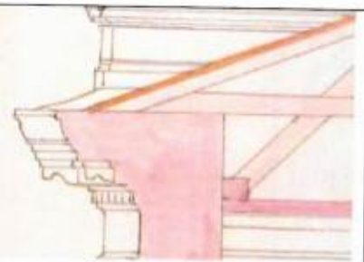
Венчающий карниз. Разрез. Проект 1886 г.
