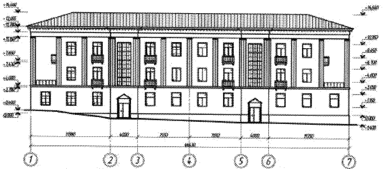
Изобр. 1. Обмерный чертеж юго-восточного (главного) фасада.
