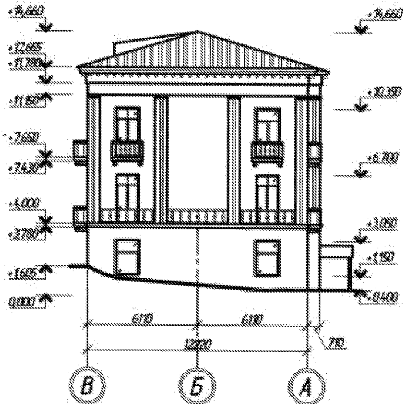
Изобр. 4. Обмерный чертеж юго-западного (торцевого) фасада
