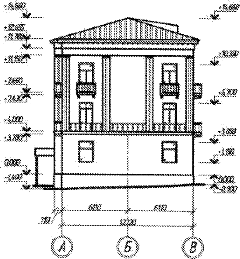
Изобр. 3. Обмерный чертеж северо-восточного (торцевого) фасада
