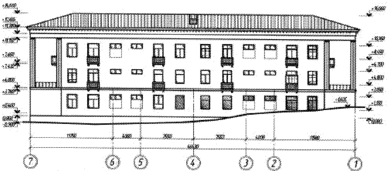
Изобр. 2. Обмерный чертеж северо-западного (дворового) фасада.
