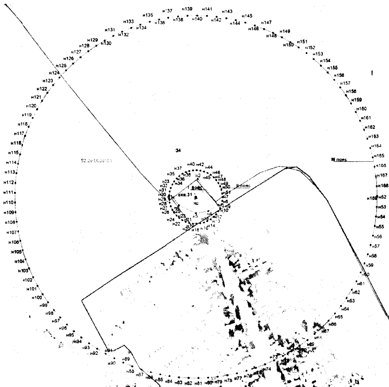
Координаты характерных точек границ первого, второго, третьего поясов ЗСО скважины № 31
