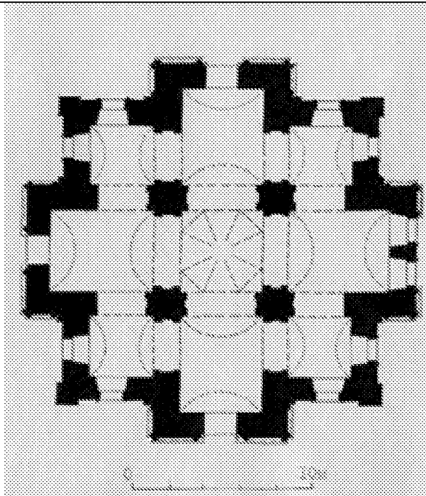
Расположение оконных и дверных проемов 1 света основного четверика
