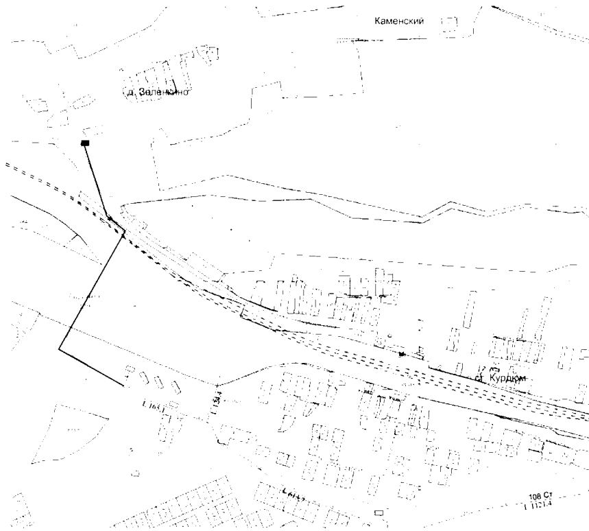
Схема 190. Газопровод межпоселковый до д. Зеленкино Татищевского района Саратовской области
