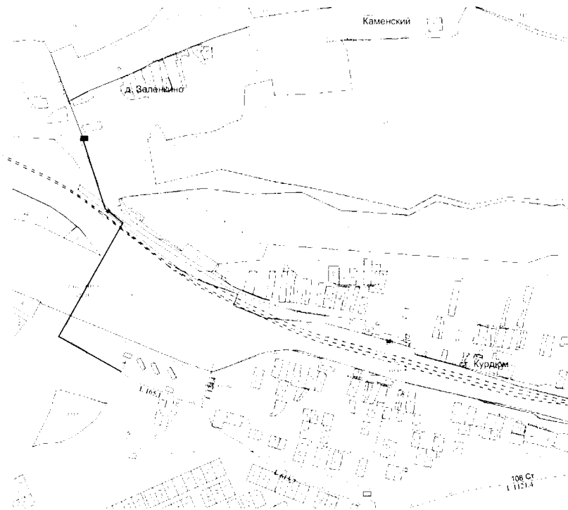
Схема 191. Распределительный газопровод в д. Зеленкино
