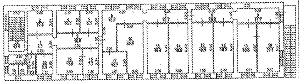
План 2 этажа
