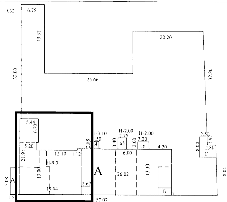
План дворового участка (план БТИ, 2010 г.) Красный прямоугольник – часть здания, постройки нач. XX в.
