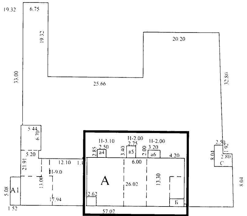
План дворового участка (план БТИ, 2010 г.) Красный прямоугольник – часть здания, постройки нач. XIX в.
