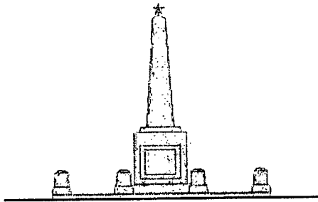
ГЛАВНЫЙ ВИД
