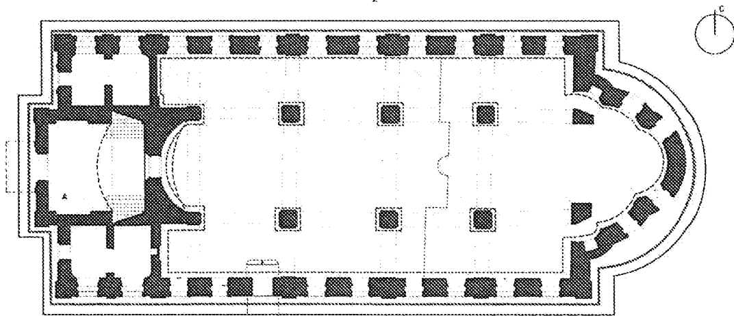
План первого этажа
