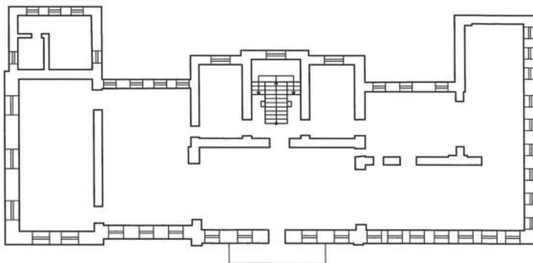
План 2-го этажа
