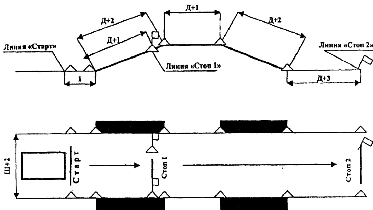
Схема 5. Остановка и трогание на подъеме
