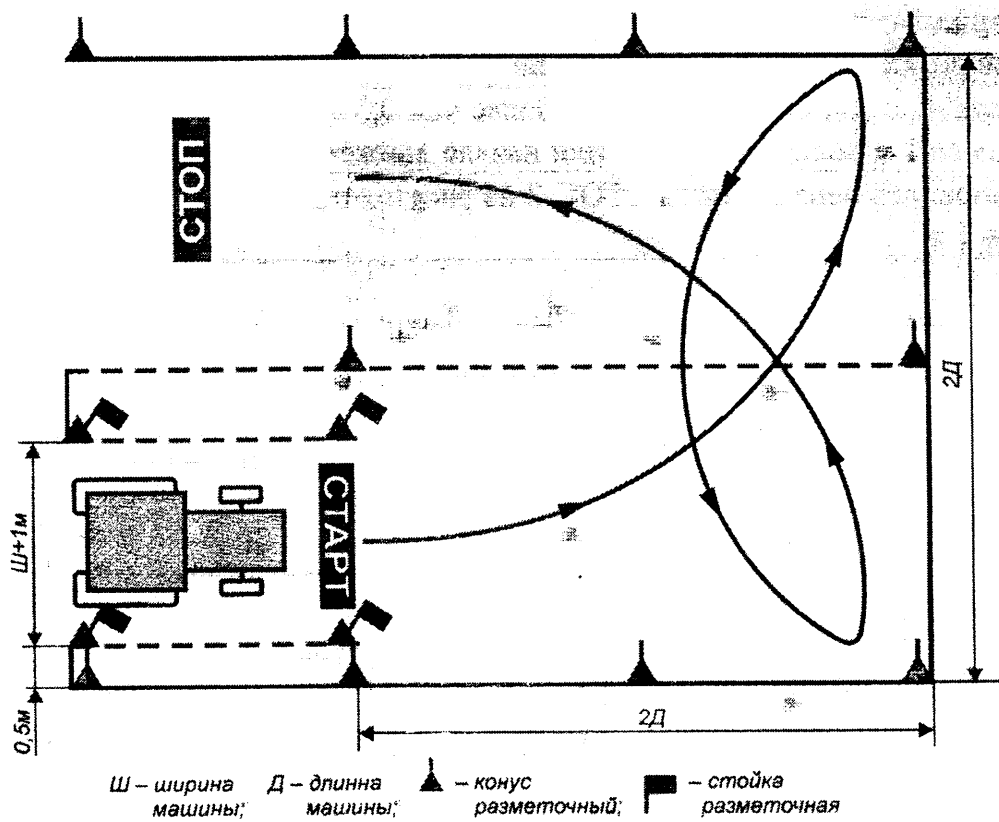
Рис. 8. Разворот маневрирование в ограниченном пространстве
