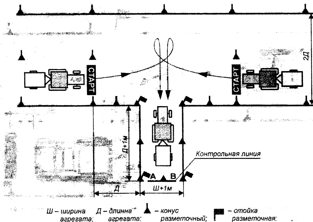
Рис. 10. Движение задним ходом, въезд в «бокс» в агрегате с прицепом
