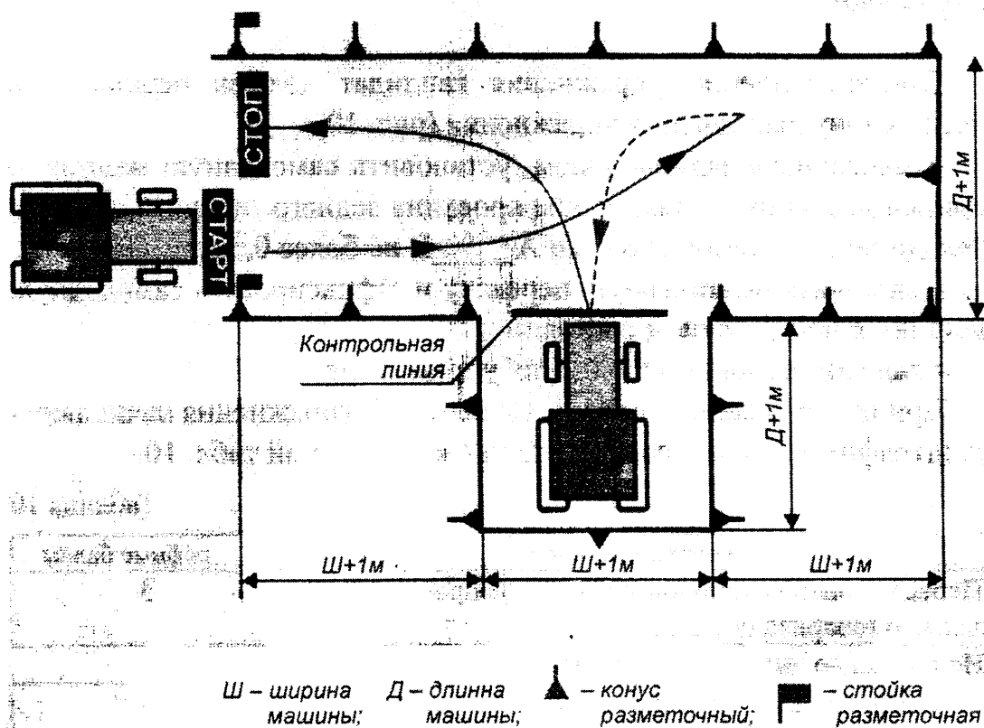
Рис. 9. Постановка самоходной машины в «бок» задним ходом
