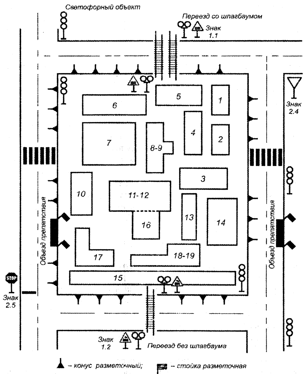
Рис. 1. Схема площадки для проведения практического экзамена
