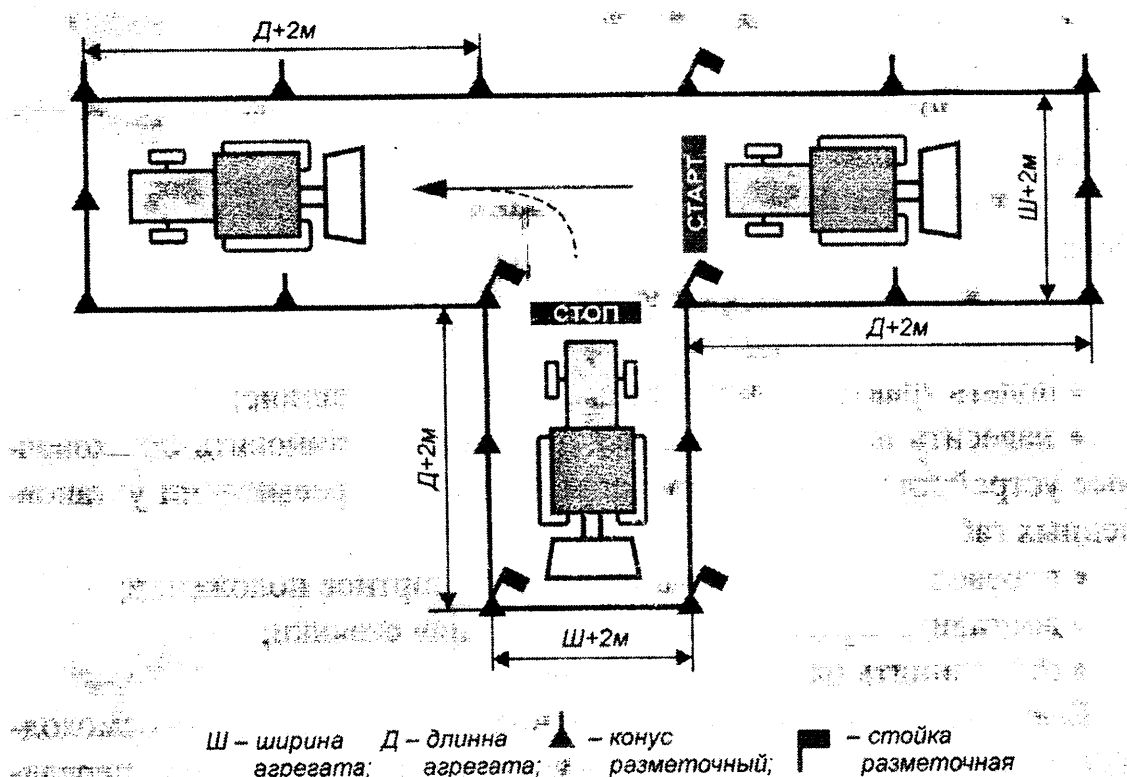
Рис. 12. Агрегатирование с навесной машиной или прицепом
