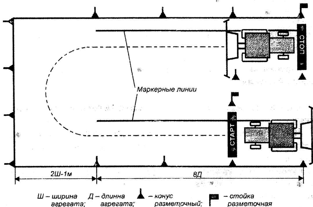
Рис. 15. Движение по маркерной или «провешенной» линии
