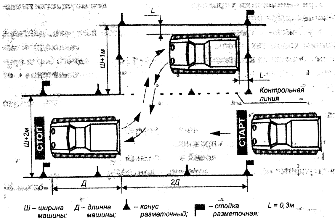
Рис. 18. Парковка СМ задним ходом и выезд с парковочного места, параллельная парковка
